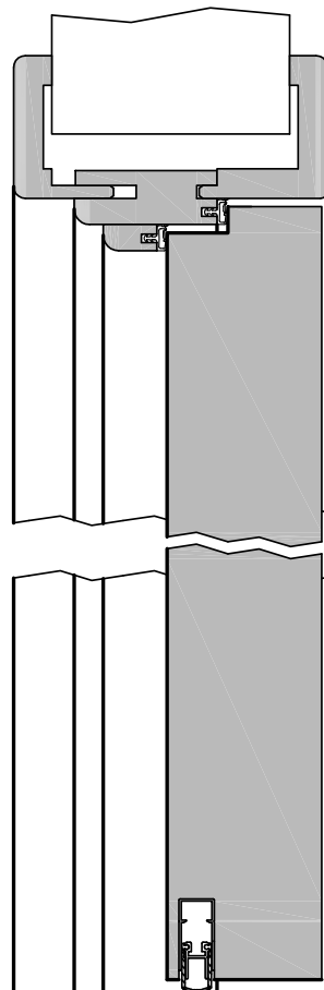
222-134-100-304-Höhenschnitt.dwg
