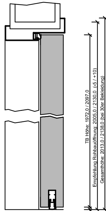
220-420-100-304-Höhenschnitt.dwg
