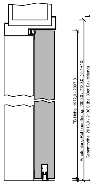
220-420-100-304-Höhenschnitt.dwg
