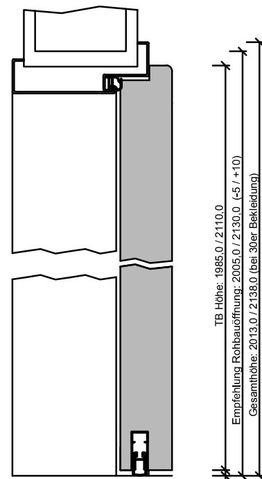
120-420-100-304-Höhenschnitt.dwg
