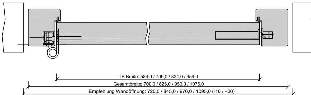
241-221-321-100-Querschnitt.dwg
