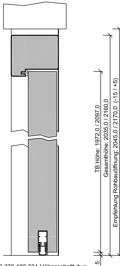
220-320-100-304-Höhenschnitt.dwg
