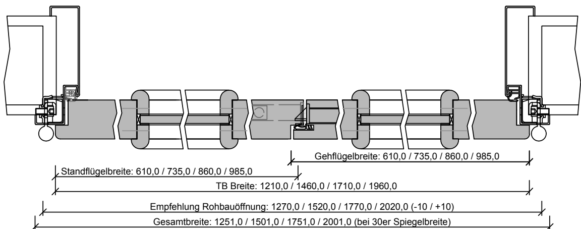
320-301-401-100-Querschnitt.dwg
