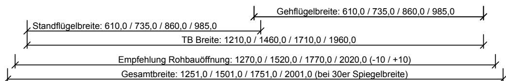
301-301-401-100-Querschnitt.dwg
