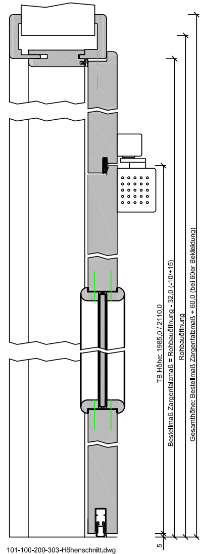
101-100-200-303-Höhenschnitt.dwg
