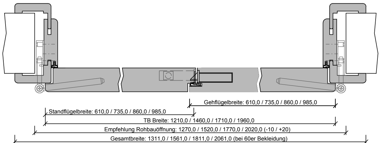
301-301-105-100-Querschnitt.dwg
