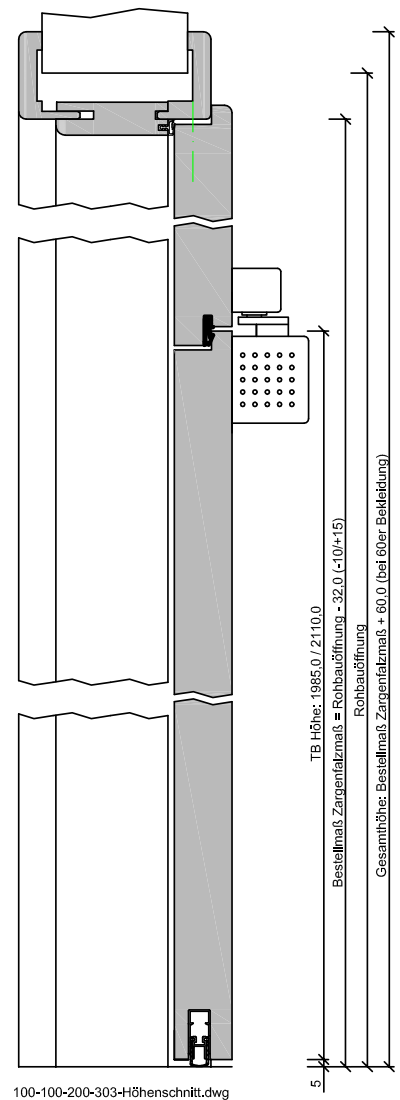
100-100-200-303-Höhenschnitt.dwg
