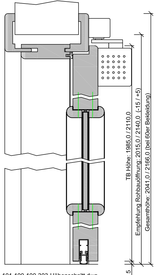
101-100-100-303-Höhenschnitt.dwg
