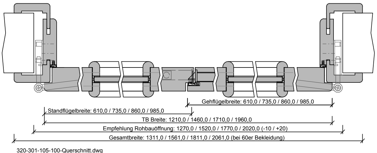
320-301-105-100-Querschnitt.dwg
