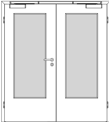
301-409-100-100_Ansicht.tcd
