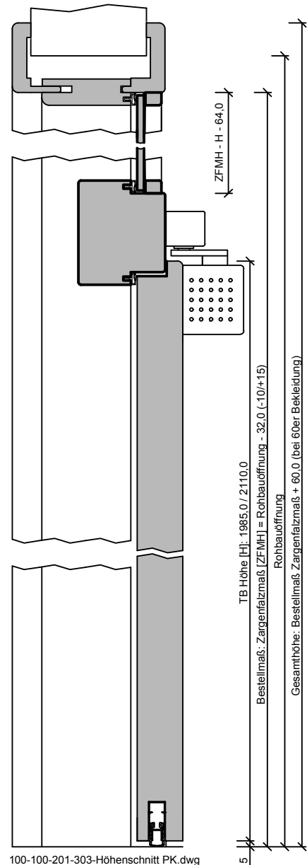
100-100-201-303-Höhenschnitt PK.dwg
