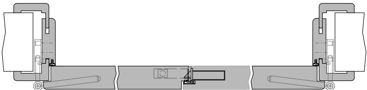
100-100-201-303-Höhenschnitt PK.dwg
