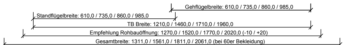
301-301-105-100-Querschnitt.dwg
