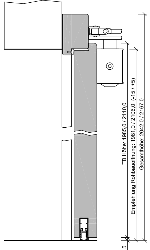
100-200-100-301-Höhenschnitt.dwg
