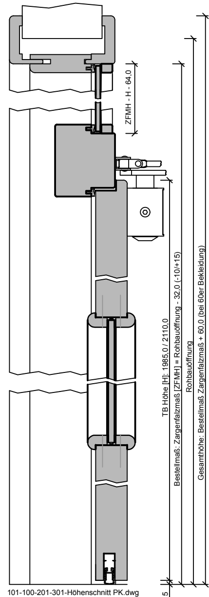
101-100-201-301-Höhenschnitt PK.dwg
