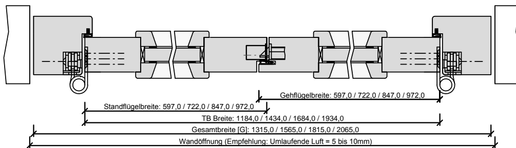
421-220-332-100-Querschnitt.dwg
