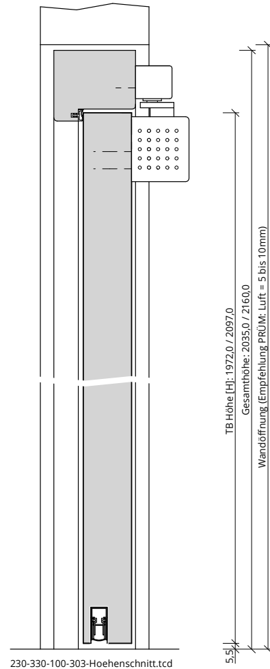
230-330-100-303-Hoehenschnitt.tcd
