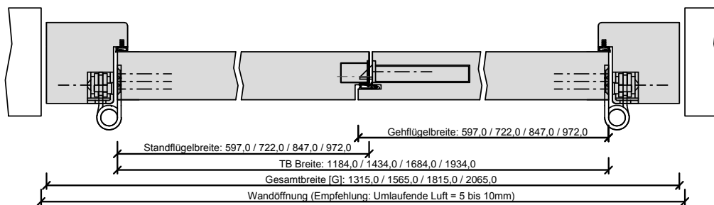
420-220-332-100-Querschnitt.dwg
