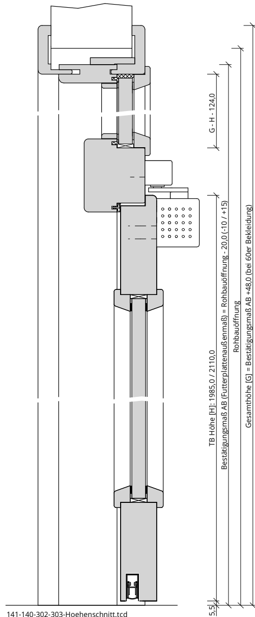
141-140-302-303-Hoehenschnitt.tcd
