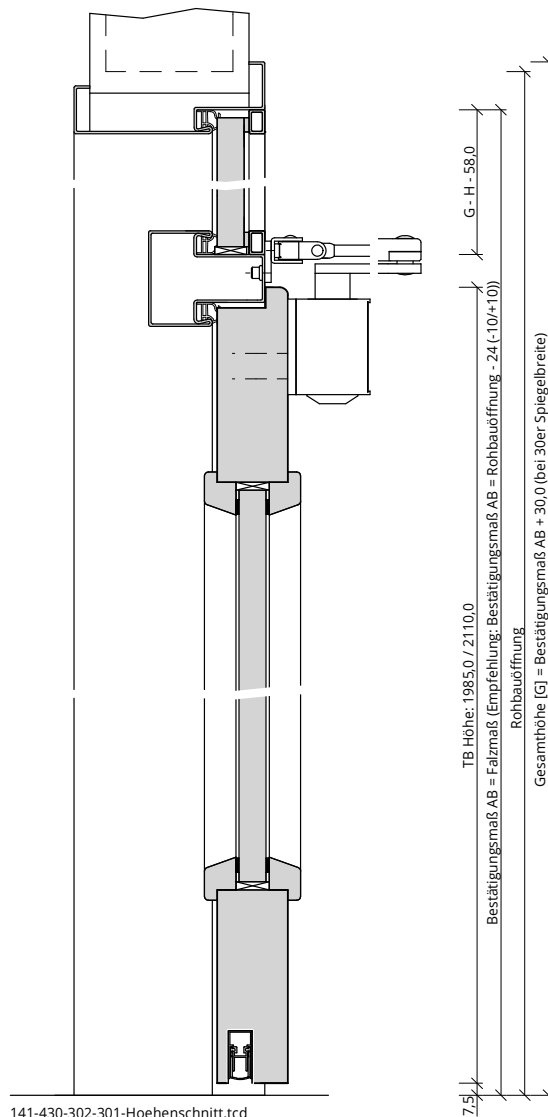
141-430-302-301-Hoehenschnitt.tcd
