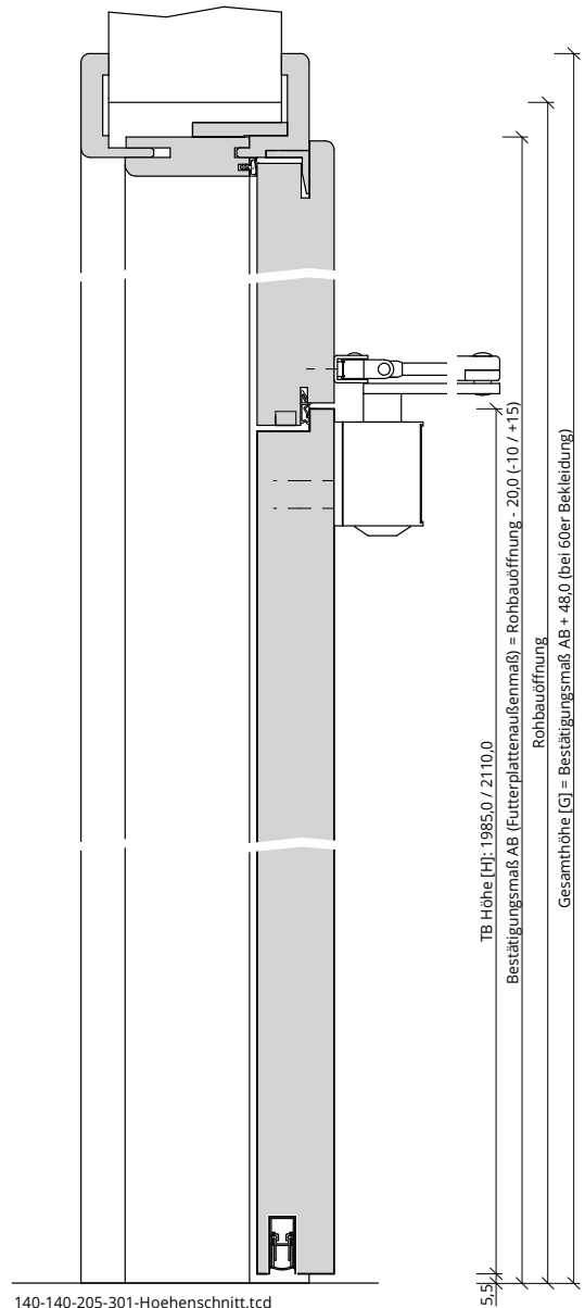
140-140-205-301-Hoehenschnitt.tcd
