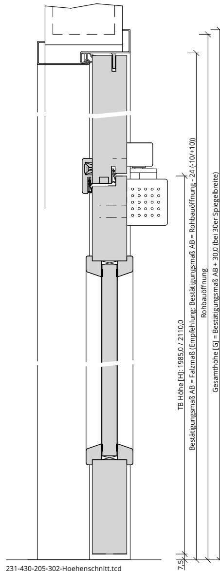
231-430-205-302-Hoehenschnitt.tcd
