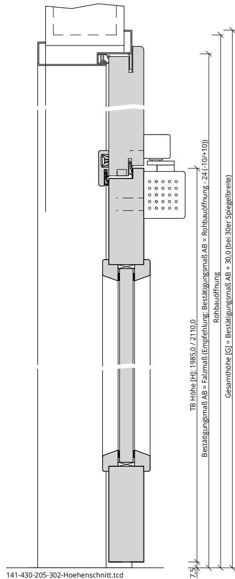
141-430-205-302-Hoehenschnitt.tcd
