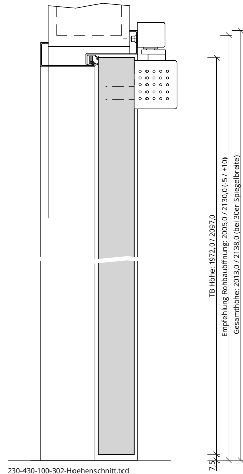
230-430-100-302-Hoehenschnitt.tcd
