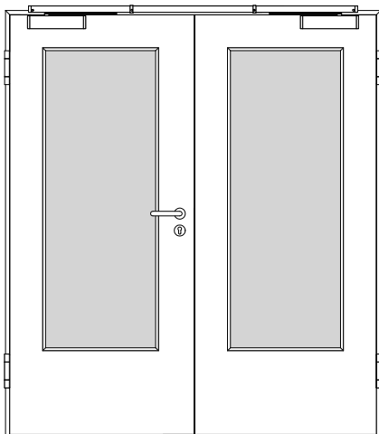
303-414-402-100_Ansicht.tcd
