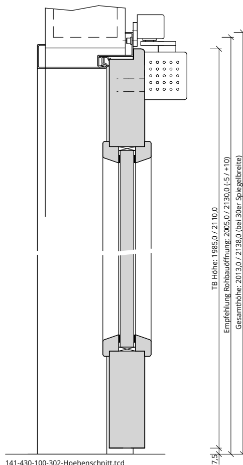
141-430-100-302-Hoehenschnitt.tcd
