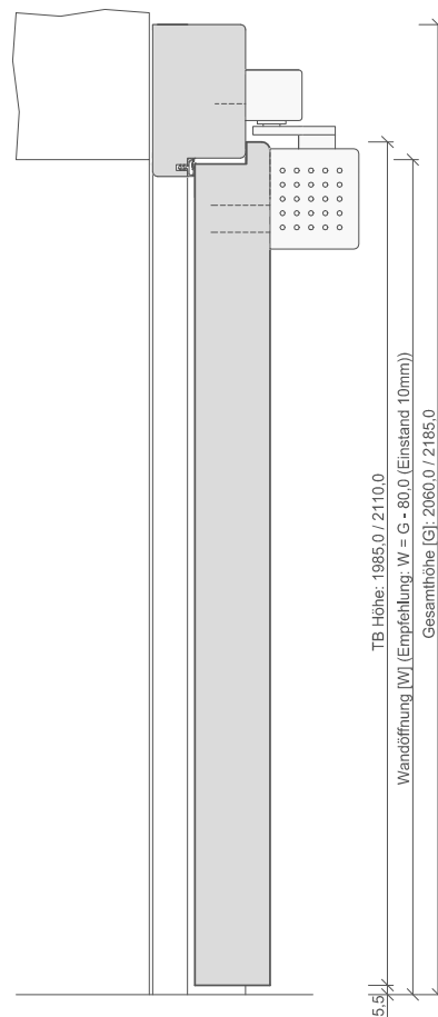
140-230-100-302-Hoehenschnitt.DWG
