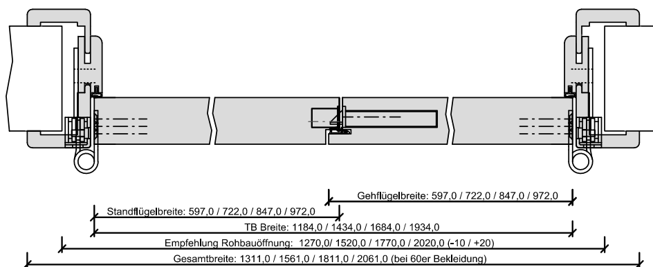
420-222-143-100-Querschnitt.dwg
