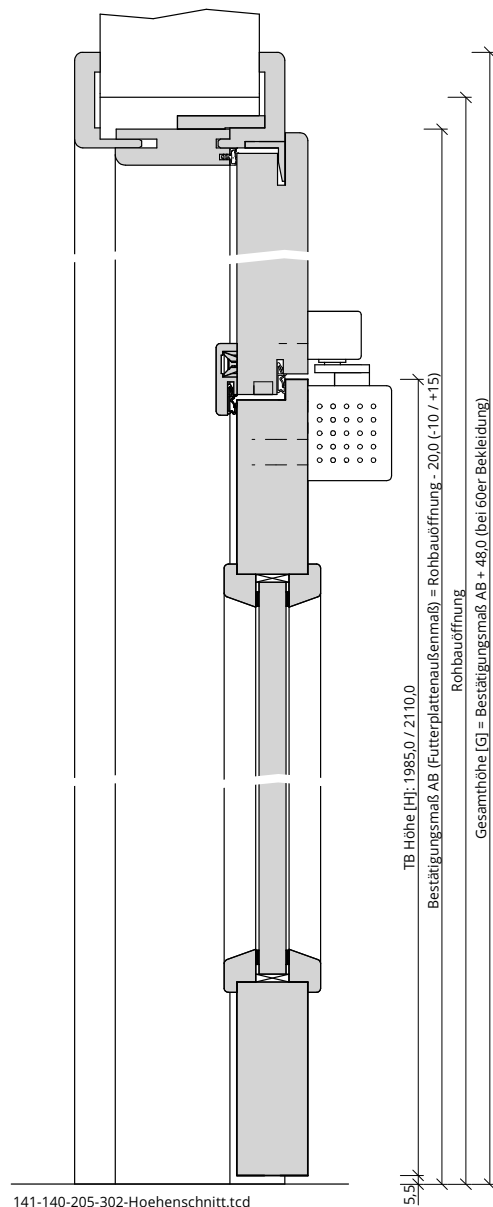
141-140-205-302-Hoehenschnitt.tcd
