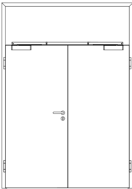
302-414-100-205_Ansicht.tcd
