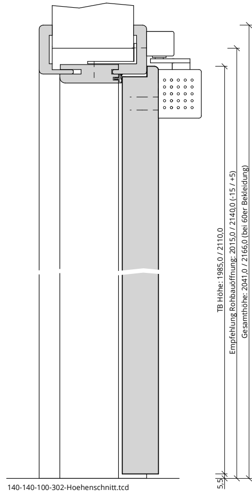
140-140-100-302-Hoehenschnitt.tcd
