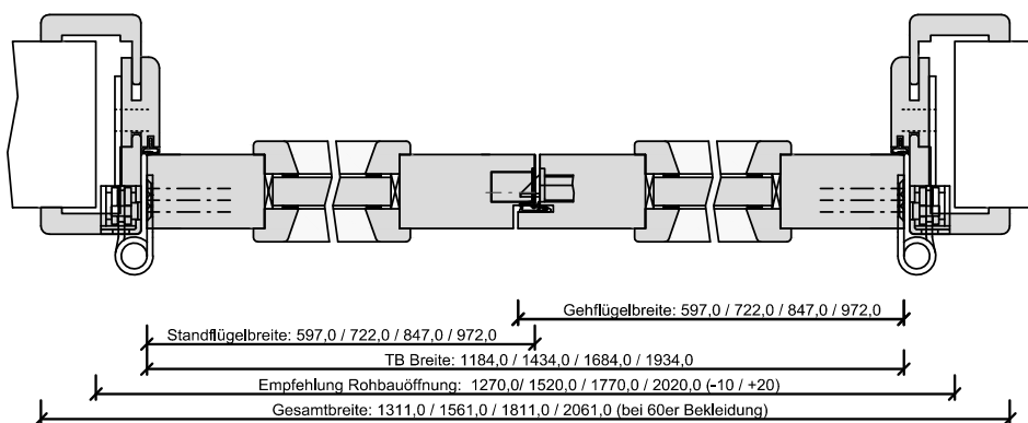
421-222-143-100-Querschnitt.dwg
