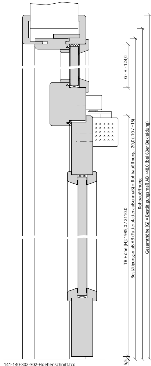
141-140-302-302-Hoehenschnitt.tcd
