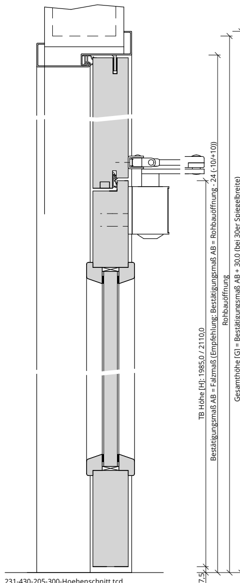
231-430-205-300-Hoehenschnitt.tcd
