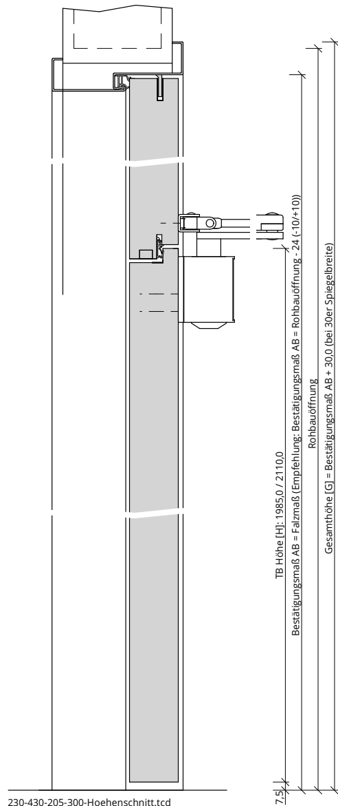
230-430-205-300-Hoehenschnitt.tcd
