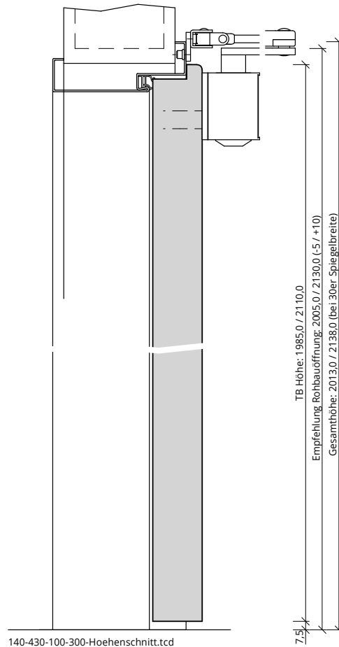
140-430-100-300-Hoehenschnitt.tcd
