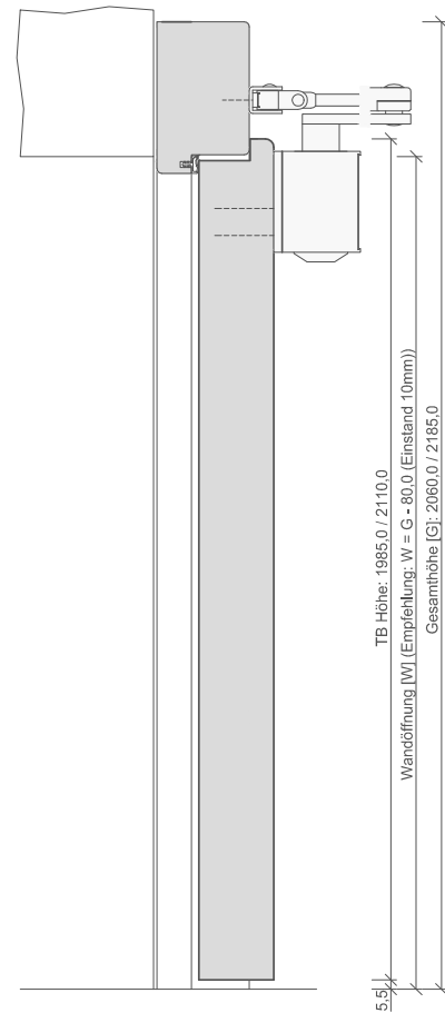
140-230-100-300-Hoeherschnitt.DWG
