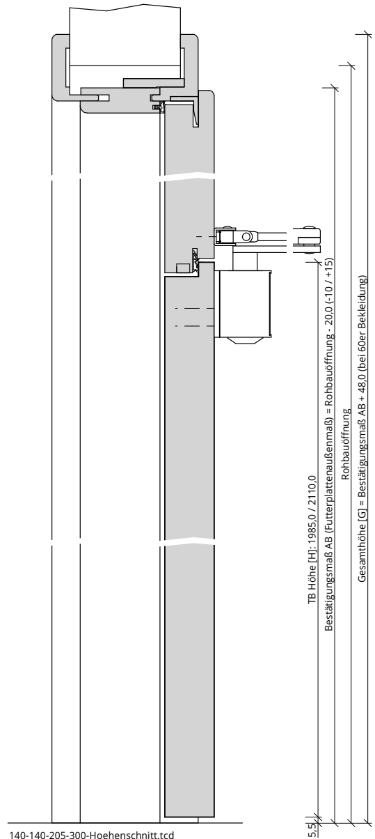
140-140-205-300-Hoehenschnitt.tcd
