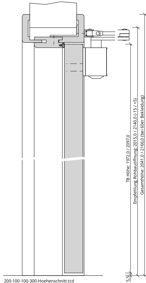
200-100-100-300-Hoehenschnitt.tcd
