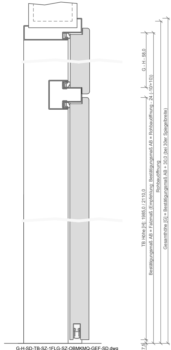
G-H-SD-TB-SZ-1FLG-SZ-OBMKMQ-GEF-SD.dwg
