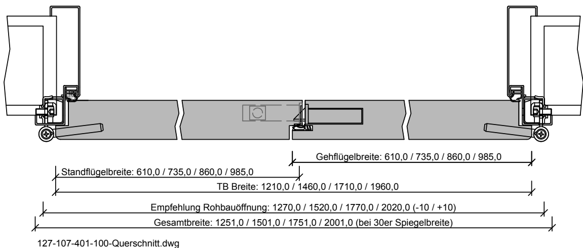
127-107-401-100-Querschnitt.dwg
