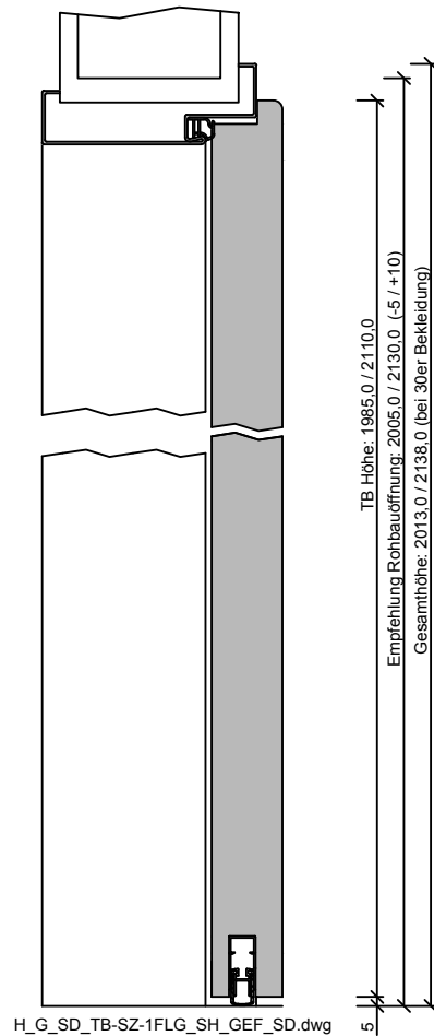
H_G_SD_TB-SZ-1FLG_SH_GEF_SD.dwg
