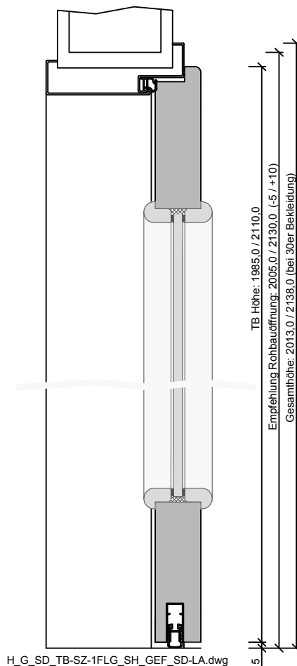
H_G_SD_TB-SZ-1FLG_SH_GEF_SD-LA.dwg
