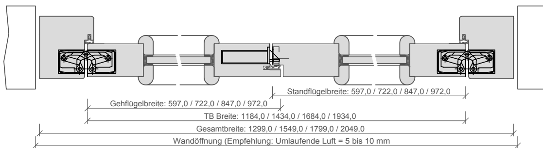
Q_RD_TB-BLO-2FLG_SH_STU_RD-40-2-LA.DWG
