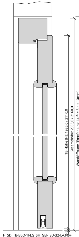
H_SD_TB-BLO-1FLG_SH_GEF_SD-32-LA.PDF
