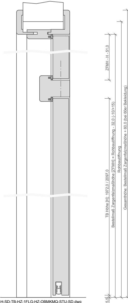
G-H-SD-TB-HZ-1FLG-HZ-OBMKMQ-STU-SD.dwg
