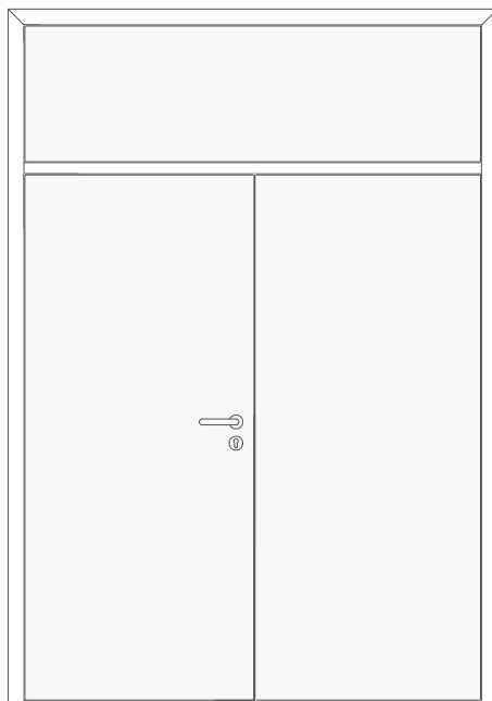
G-A-SD-TB-HZ-2FLG-HZ-OBMKMQ-STU-SD.dwg
