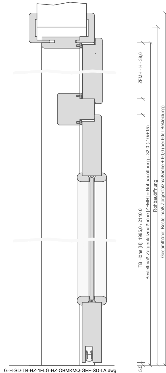
G-H-SD-TB-HZ-1FLG-HZ-OBKMQ-GEF-SD-LA.dwg
