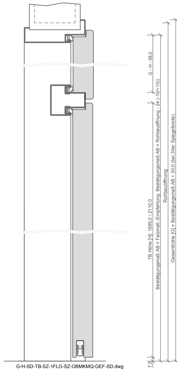
G-H-SD-TB-SZ-1FLG-SZ-OBMMQ-GEF-SD.dwg
