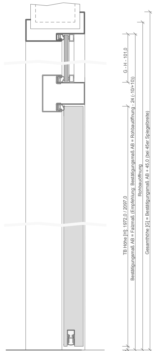
G-H-SD-TB-SZ-1FLG-SZ-WF2-OLMKMQ-STU-SD.dwg
