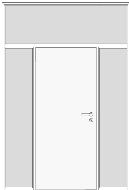
G-A-SD-TB-SZ-1FLG-SZ-WF2-OLMKMQ-STU-SD.dwg
