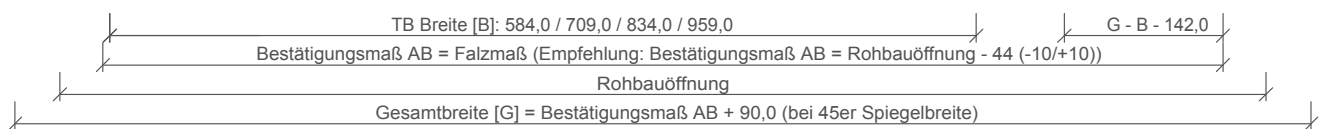
G-Q-SD-TB-SZ-1FLG-WF1-STU-SD.dwg
