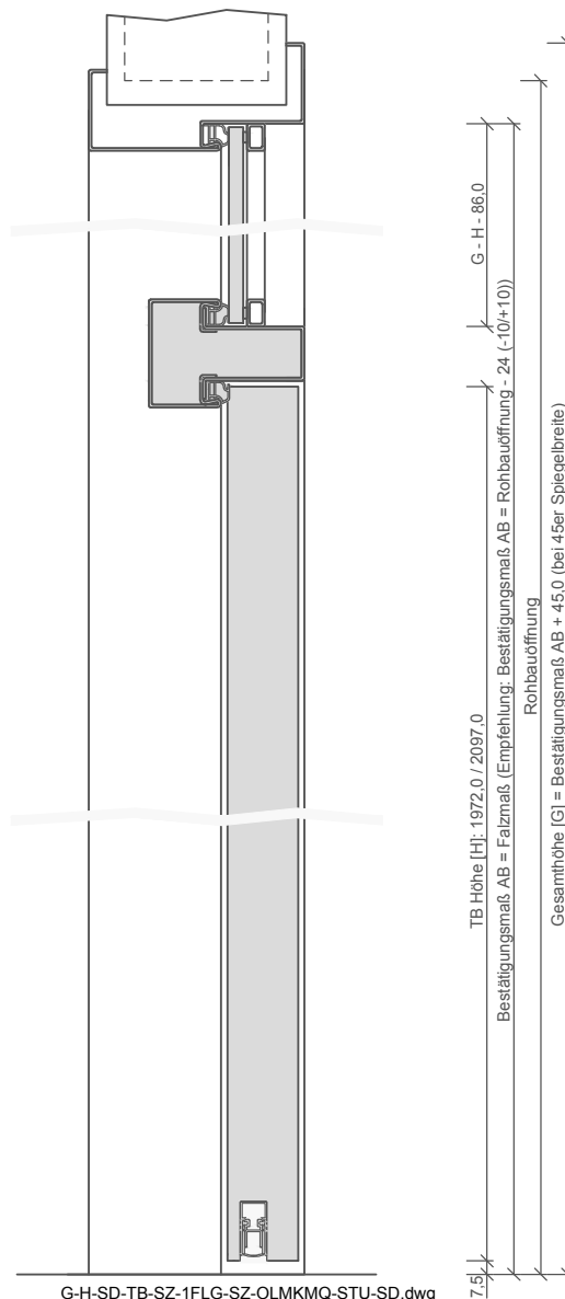
G-H-SD-TB-SZ-1FLG-SZ-OLMKMQ-STU-SD.dwg
