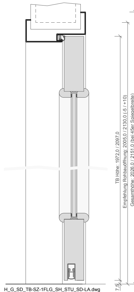
H_G_SD_TB-SZ-1FLG_SH_STU_SD-LA.dwg
