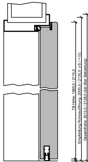
105-400-100-304-Höhenschnitt.dwg
