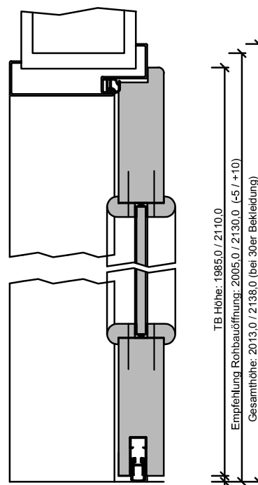
110-400-100-304-Höhenschnitt.dwg
